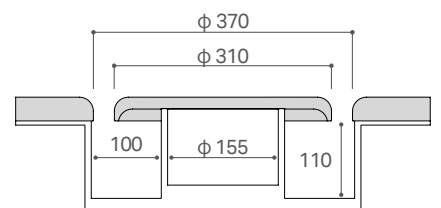
④ ワイヤリングシステム寸法
