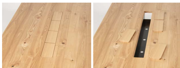
(参考写真) ソリッドテーブル用ワイヤリングシステム (通線カバー 4 枚タイプ)
